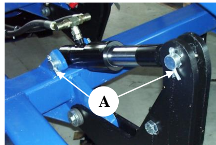
NSH stenudløser
