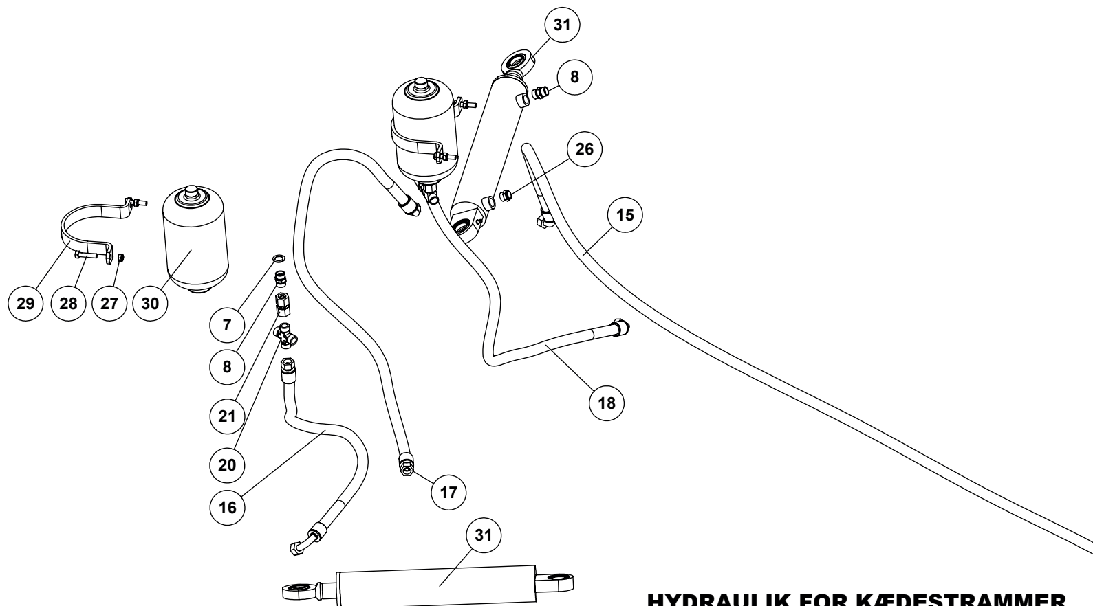
HYDRAULIK FOR KÆDESTRAMMER POWERCHAIN 1200 HYDRAULIK FÜR KETTENSPANNER HYDRAULICS FOR CHAIN TENSIONERS HYDRAULIQUE POUR TENDEURS DE CHÂÎNE 68219
