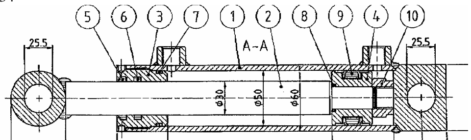
Vérin 50/30-150
