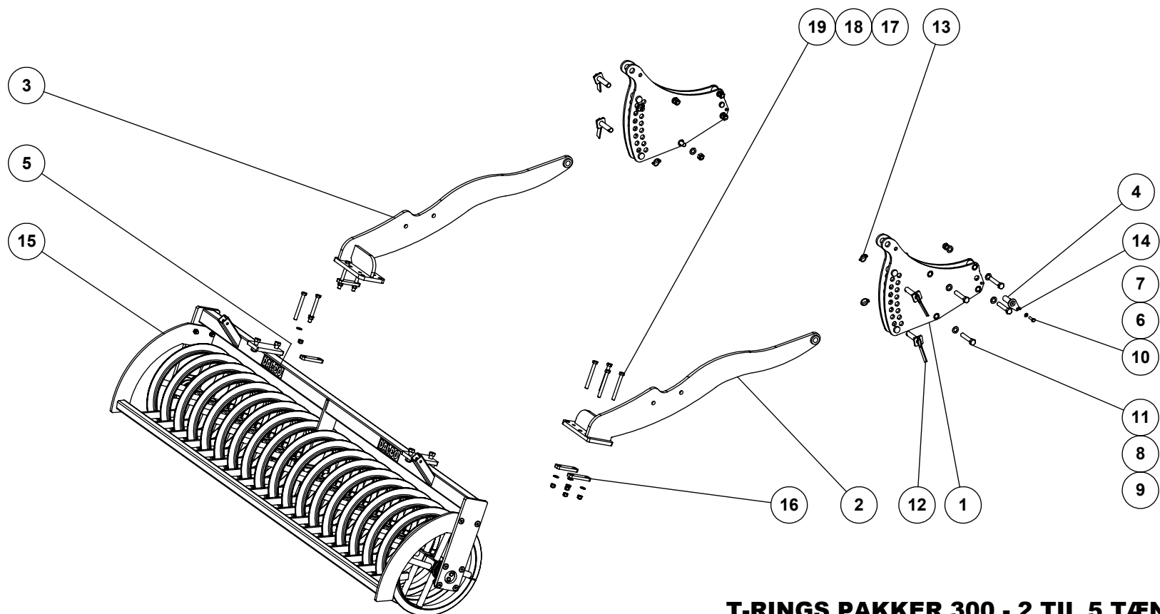
T-RINGS PAKKER 300 - 2 TIL 5 TÆNDER SUBSOILER NÄCHLAUFER ROLLER, T-RING TRaine, ANNEAU-T 82037
