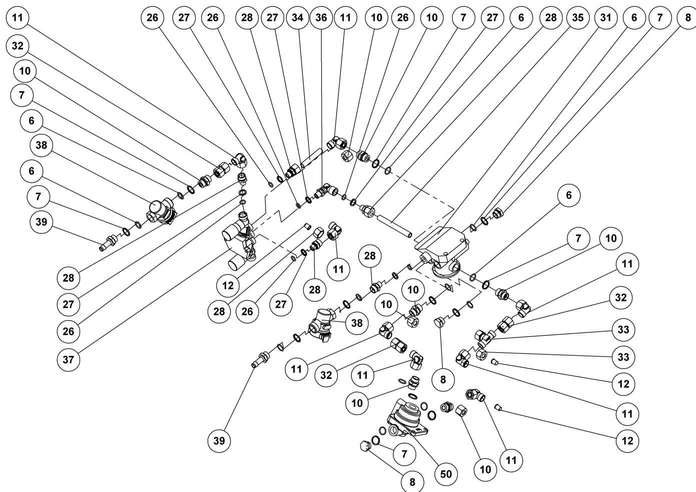
TRYKLUFTEBREMSE EXCL. HJUL OG LYS - 6 HULS NAV POWERROLL 1030/1230
