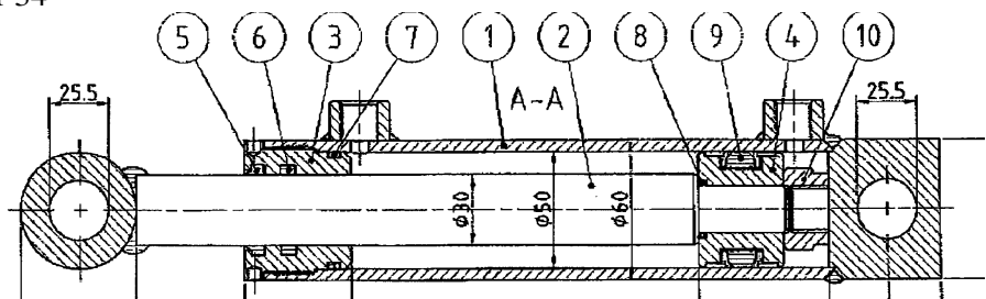
Zylinder 50/30-150
