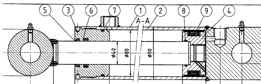
Zylinder 80/40-350 (91805)
