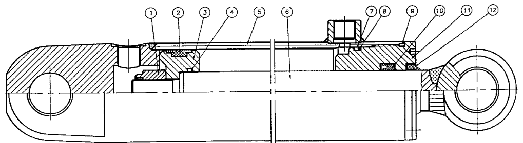
Zylinder 70/30-205
