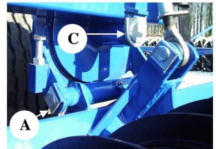
Rechte Seite
